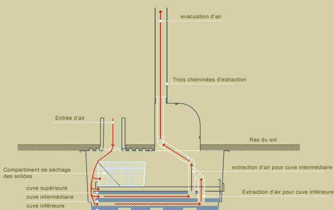
Système à 3 cuves avec ventilation renforcée
